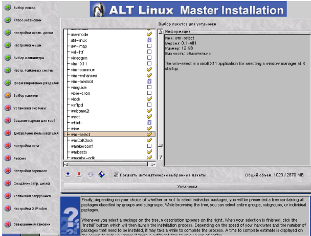
Рисунок 9.12. Загрузка списка пакетов
