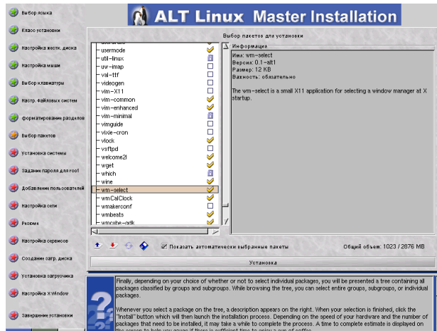
Рисунок 9.11. Индивидуальный выбор пакетов
